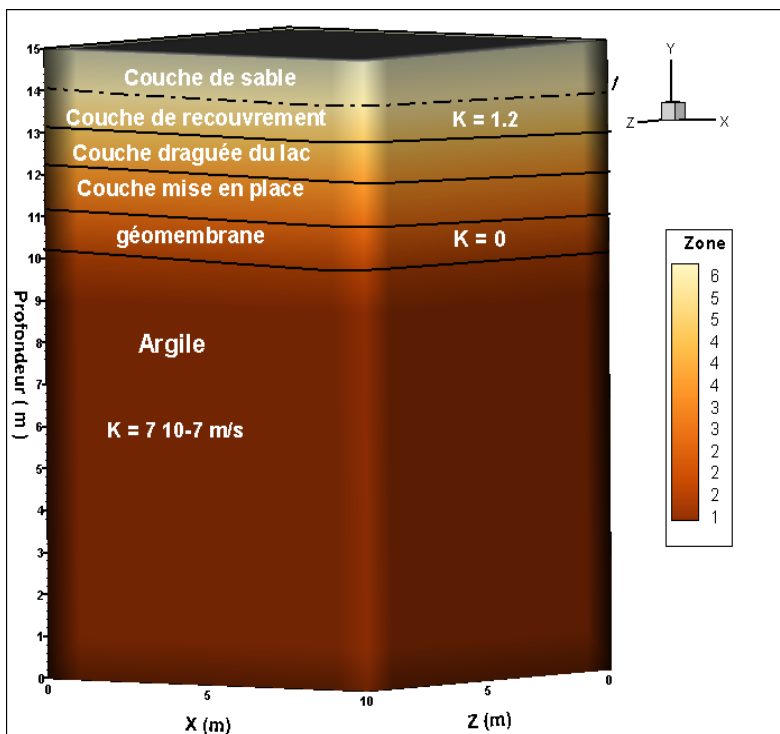
Figure 2 : Schéma du modèle conceptuel 3D simulé avec HydroGeosphere.
