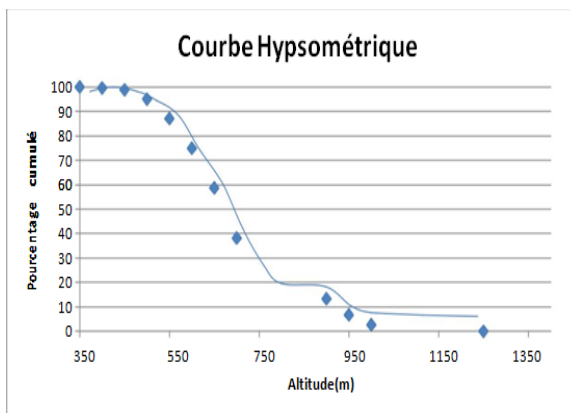
Figure n° 2 : Courbe hypsométrique du bassin versant oued Siliana
