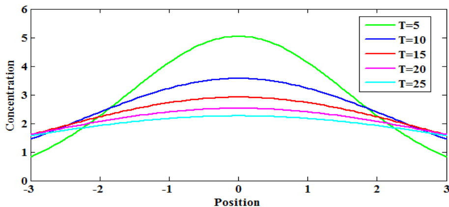
Fig. 2 - Variation de la concentration d' air en fonction de la position
