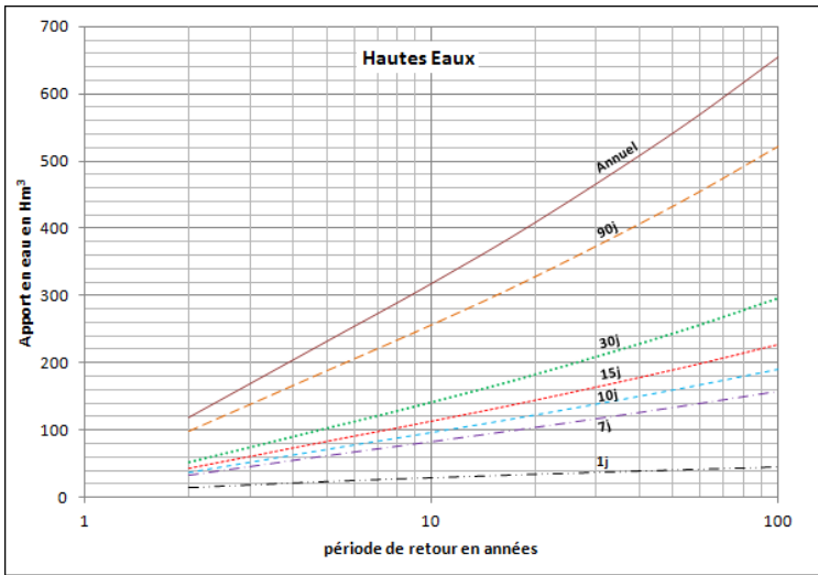
Fig. 2. Courbes QdF de l'oued Kébir-Ouest à Ain Charchar
