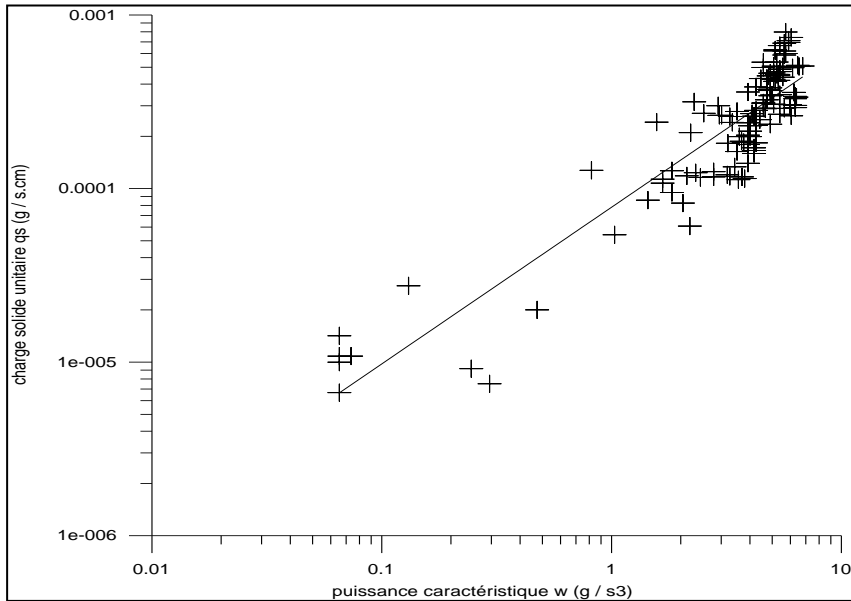
Fig. 5. Charge solide et puissance du courant dans les essais expérimentaux.
