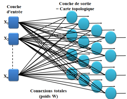
Fig. 2 - Schéma d'une carte de Kohonen
