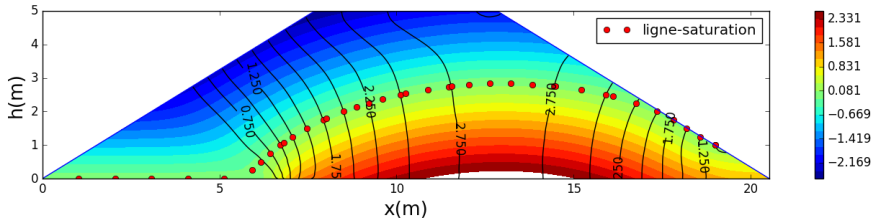
Figure 6. Ligne de saturation dans un barrage homogène à drain horizontal après 30 heures de vidange
