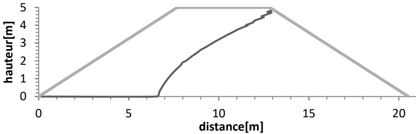
Figure 2. Ligne de saturation dans un barrage homogène à drain horizontal (régime permanent)
