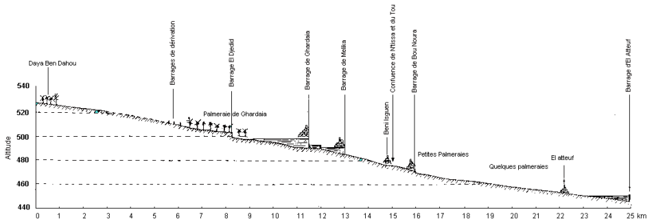
Figure 2 : Coupe géomorphologique schématique de la vallée de M'Zab
