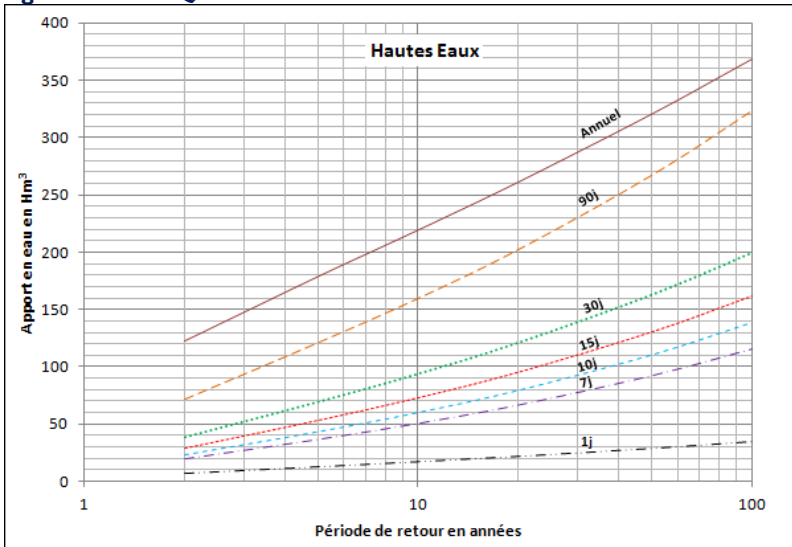
Fig. 3. Courbes QdF de l'oued Rhumel à Grarem
