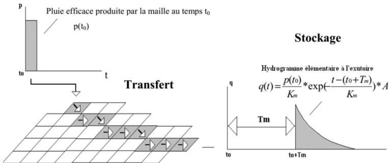
Figure 3 : Représentation de la fonction de transfert sous MERCEDES [17]
