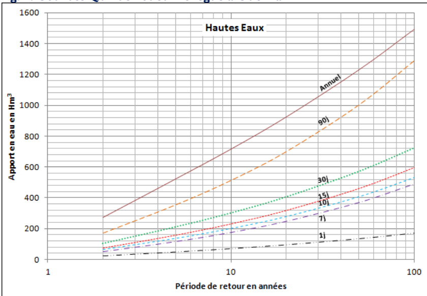
Fig. 5. Courbes QdF de l'oued Seybouse à Mirbeck
