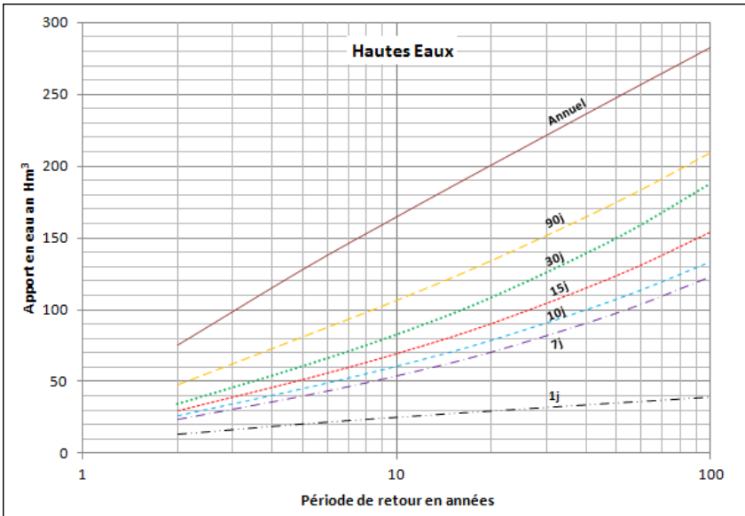
Fig. 4. Courbes QdF de l'oued Mellegue à Ouenza
