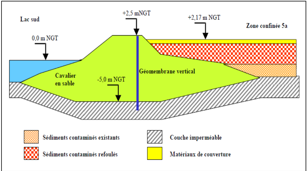
Figure 1 - Système de confinement mis en place sur les berges ouest du lac (Ben Charrada et Jouini, 2002).
