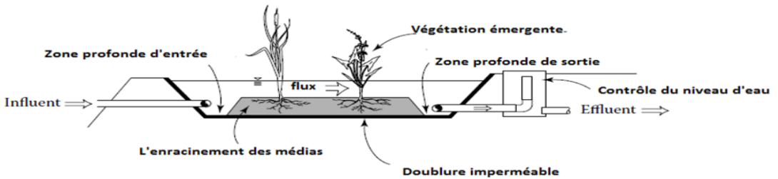
Figure 1. Éléments de base d'un jardin filtrant avec écoulement a surface libre [4].
