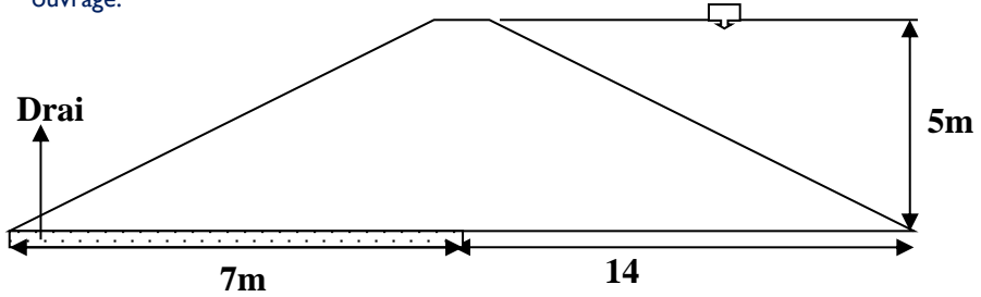
Figure 1. Barrage homogène isotrope à tapis filtrant
