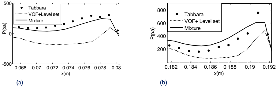
Fig. 3 – profils de pression (a) le long de la 3 ème marche (b) le long de la 12 ème marche
