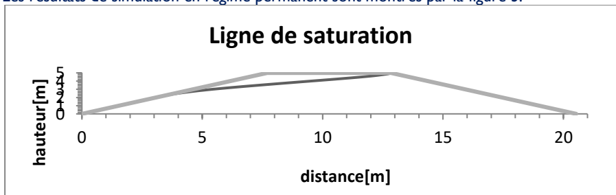
Figure 3. Ligne de saturation dans un barrage homogène (régime permanent)
