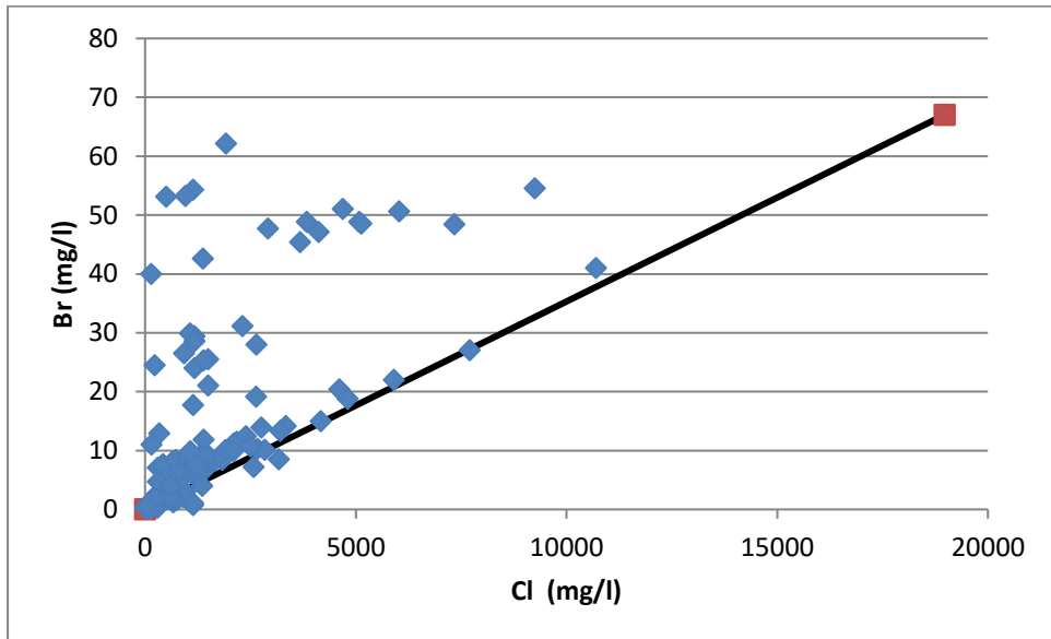
Figure 3. Corrélation entre le Brome et le chlore.
