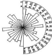
Figure 1 : Rosace directionnelle du champ de fracturation obtenue dans la zone d'étude
