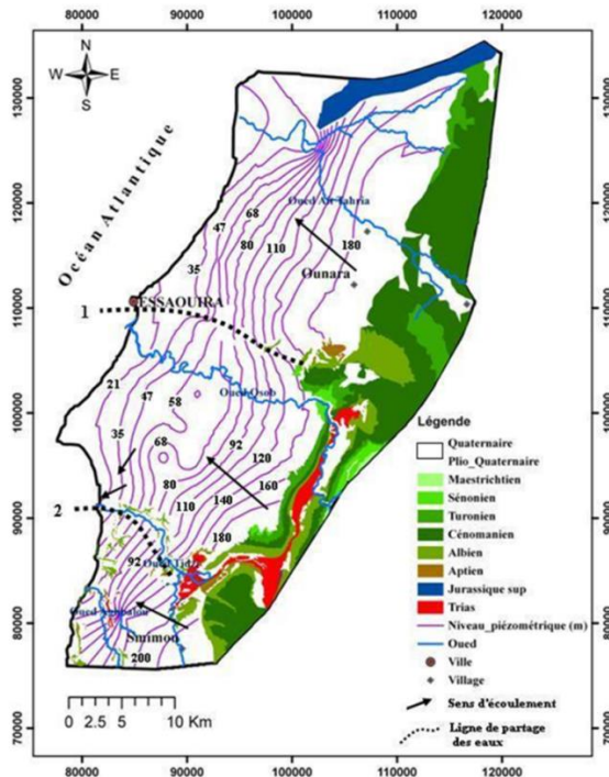
Fig. 6 - Carte piézométrique du réservoir plio-quaternaire (septembre 2013).
