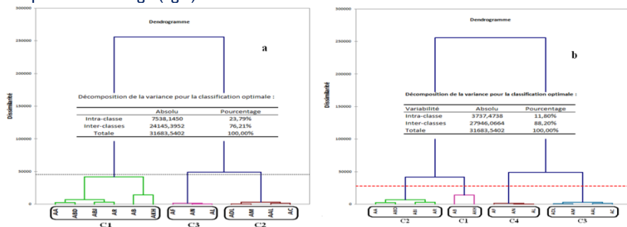
Fig. 6. Classification des sources du complexe structural de l'Edough: a- Partition en 3 classes ; b- Partition en 4 classes
