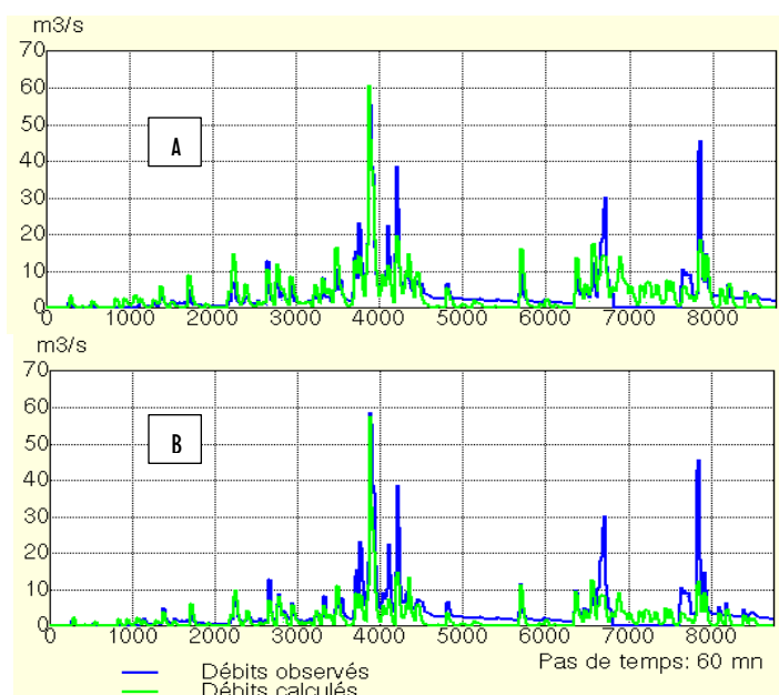
Figure 5 : Hydrogrammes annuels observés et observés à la Bété en phase de : A-) calage et B-) validation (2017)
