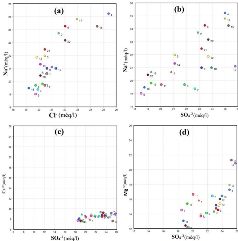
Fig.5. Relations entre les éléments majeurs: (a) Navs. Cl ; (b) Navs. SO 4 ; (c) Ca vs. SO 4 ; (d) Mg vs. SO 4 .
