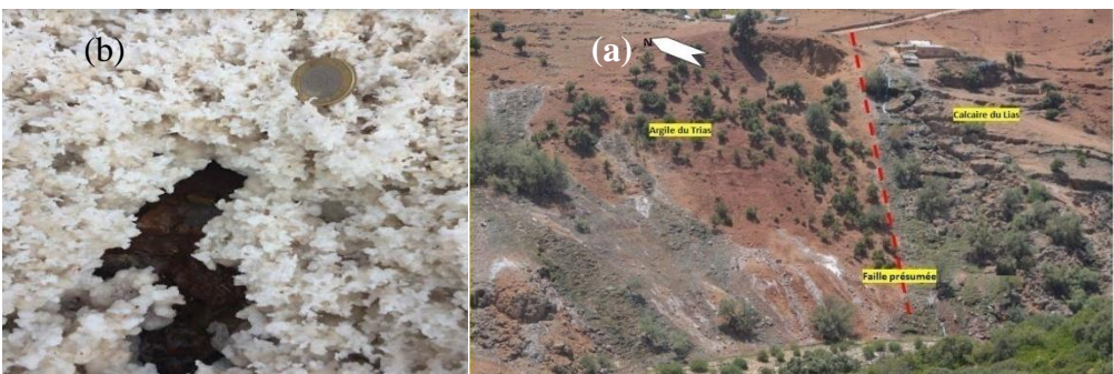
Figure 4 – photo d'un accident mettant en juxtaposition les calcaires lités du Lias et les argiles du Trias, et les écoulements salés dans les argiles triasiques (a), photo de dépôts de sels s'accumulant sur les argiles du Trias (b). (Cliché T.Amine 20/08/2017).
