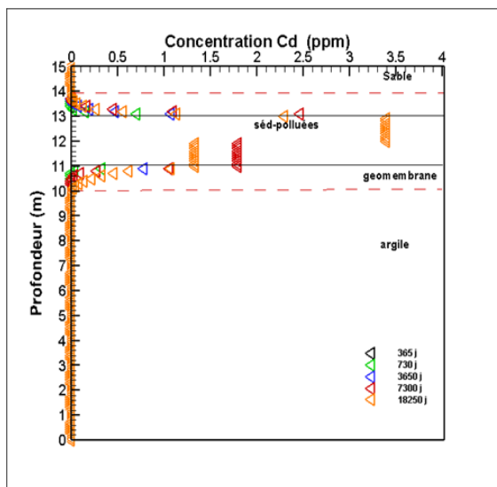
Figure 3 : Concentration en ppm du Cd en fonction du temps et de la profondeur
