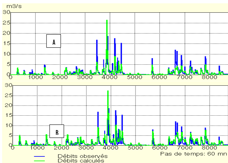
Figure 7 : Hydrogrammes annuels observés et calculés à la Djibi en phase de : A-) calage et B-) validation (2017)
