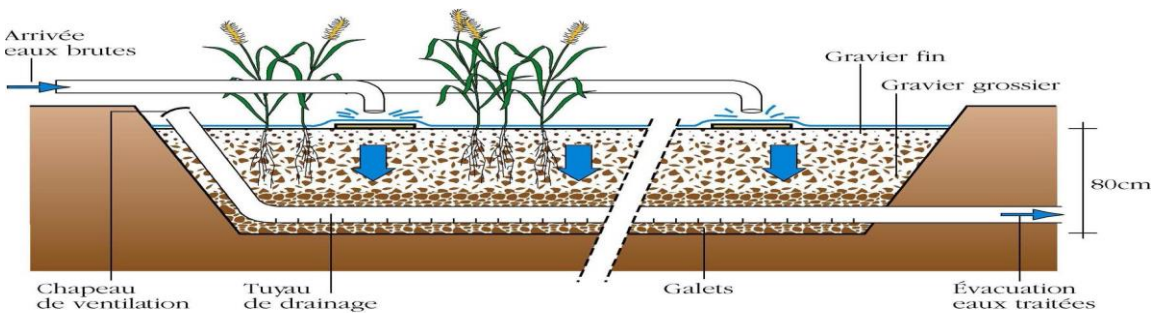
Figure 3 .coupe transversale schématique d'un filtre a ecoulement vertical [7] .
