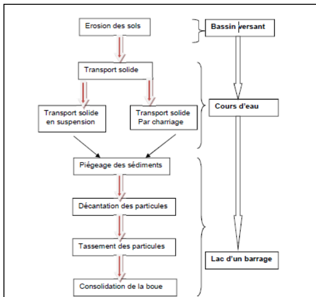
Fig. 1. Processus d'envasement d'un barrage Réservoir (Remini, 1990)
