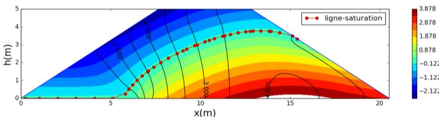
Figure 5. Ligne de saturation dans un barrage homogène à drain horizontal après 10heures de vidange
