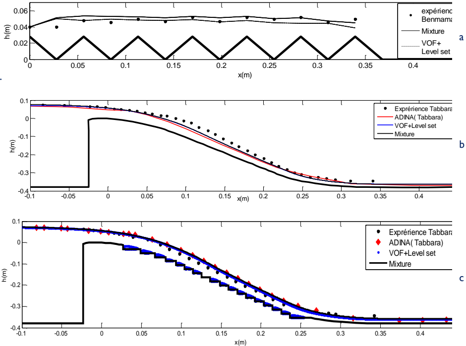
Fig. 2 – profils de la surface libre (a) canal à marches d'escalier horizontal, (b) coursier lisse à forte pente, (c) coursier à marches d'escalier à forte pente
