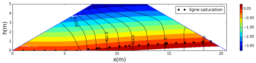
Figure 7. Ligne de saturation dans un barrage homogène à drain horizontal après 10 jours de vidange
