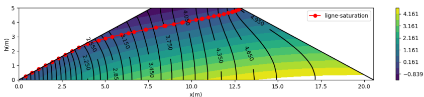
Figure 4 lignes d'équipotentiels et lignes d'équipressions (régime permanent)
