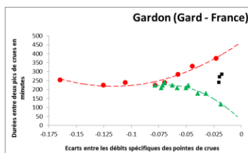
Fig. 2 - Relation entre les écarts des débits spécifiques à Ners et à Russan et le décalage temporel des pointes de crues
