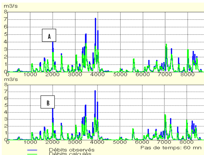
Figure : 6 Hydrogrammes annuels observés et calculés à la Djibi en phase de : A-) calage et B-) validation. (2016)
