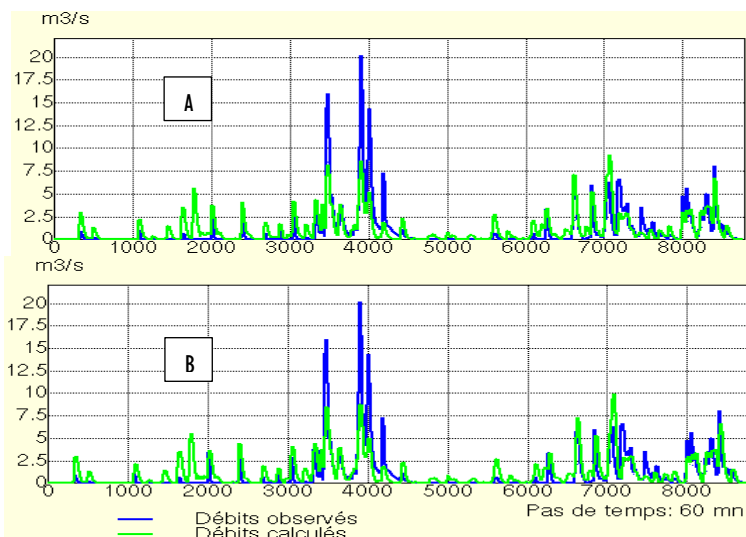
Figure 4 : Hydrogrammes annuels observés et calculés à la Bété en phase de : A-) calage et B-) validation(2016)
