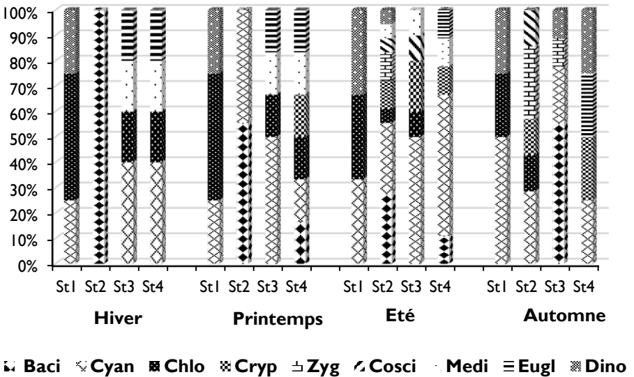
Fig. 5 - Contribution relative (%) des groupements phytoplanctoniques dans le Béni Haroun (Abréviations: Cryp—Cryptophyceae; Cyan—Cyanophyceae; Baci—Bacillariophyceae; Chlo—Chlorophyceae; Eugl—Euglenophyceae; Cosci—Coscinodiscophyceae; Dino—Dinophyceae; Medi—Mediophyceae; Ulvo—Ulvophyceae; Zyg—Zygnematophyceae)
