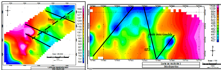
Fig. 2- Carte de résistivité apparente des site 1 et 2
