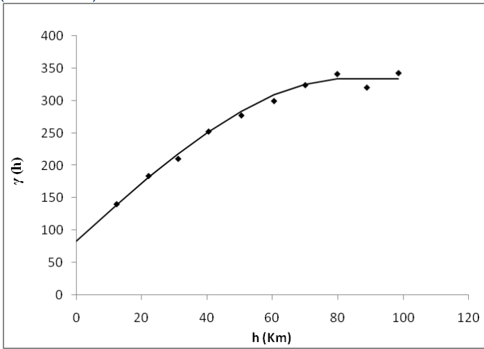
Figure 3. Variogramme de la fracturation tous azimut, Ajustement à un modèle sphérique
