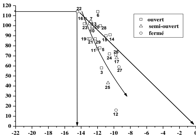
Fig n° 1 : Relation \delta^{13}\text{C} / \text{a}^{14}\text{C} dans les eaux des systèmes karstiques des Monts de Tlemcen
