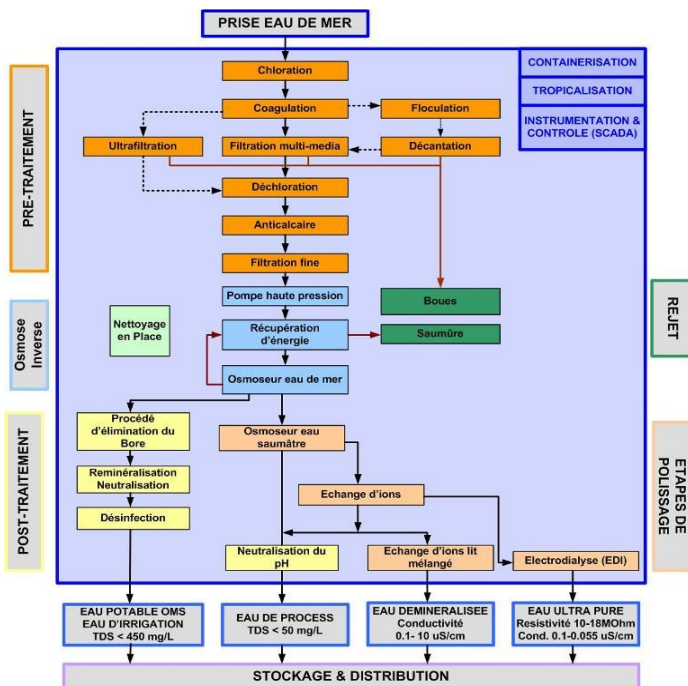
Schéma N°1 : « Principales étapes dans le procédé de dessalement »
