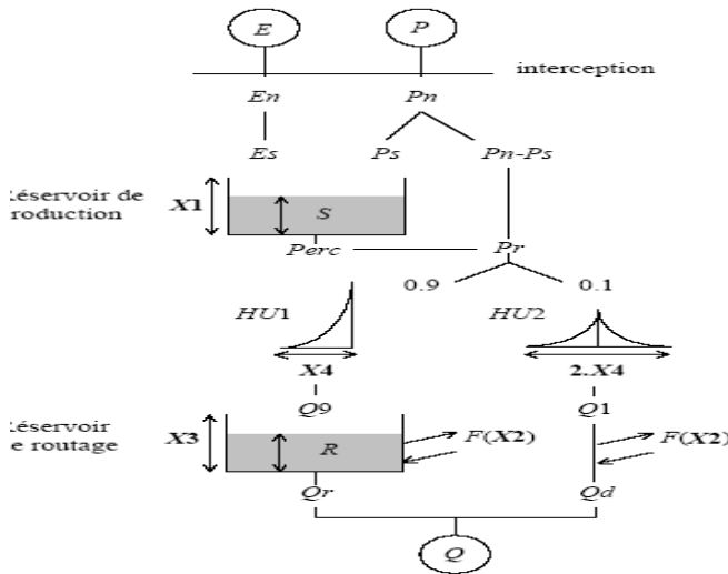
Figure II. Structure générale du modèle GR4j [17]
