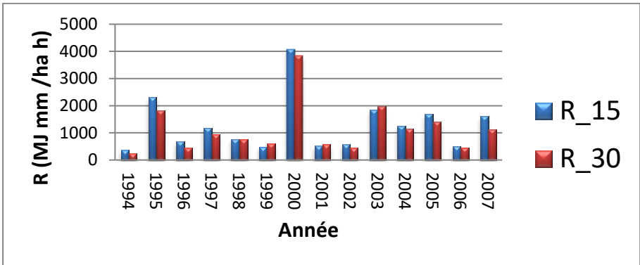
Fig. 3. Variation annuelle de l'érosivité calculée pour l'intensité maximale 15' et 30'.
