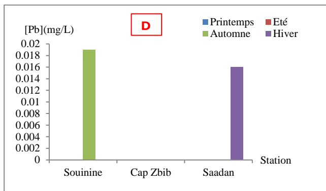
Fig. 2 - Variation spatio-temporelle des teneurs en Aluminium (A), Chrome (B), admium (Cd) et Plomb (Pb) dans les eaux des trois sources étudiées (Printemps 2012-Hiver 2013).
