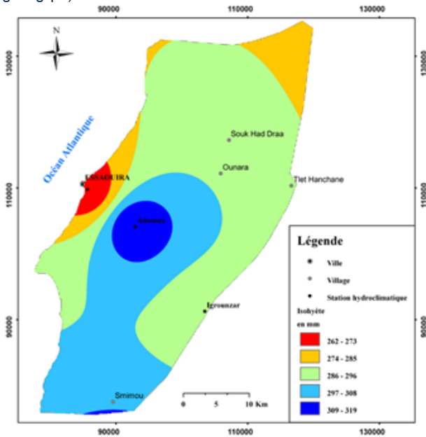
Fig. 2 - Carte du potentiel pluviométrique de la zone côtière d'Essaouira (1990-2015).
