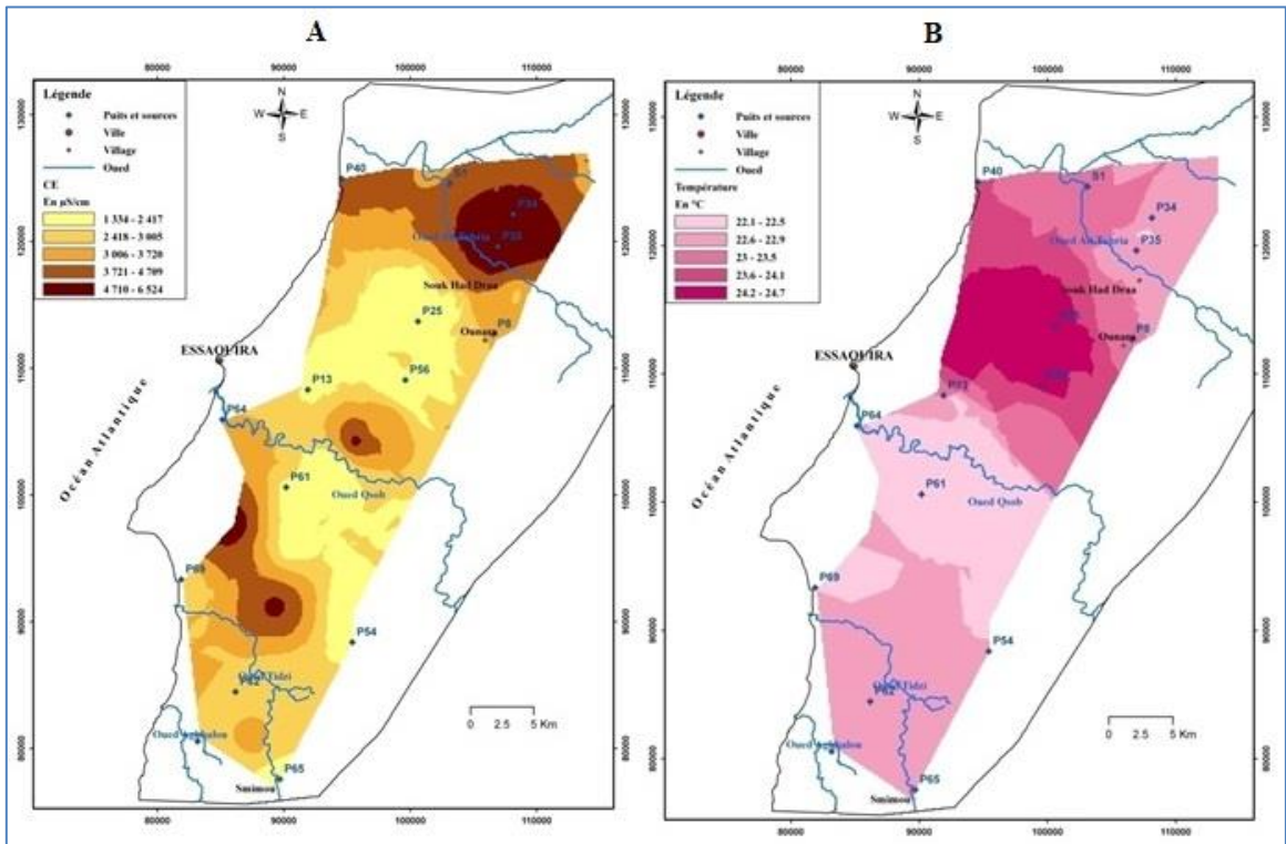
Fig. 7 – Cartes des paramètres physiques des eaux de la nappe côtière d'Essaouira (A : La répartition de la conductivité électrique. B : La répartition de la température des eaux sous terrains).
