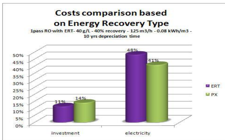
Graph N° 2 : le coût de l'électricité et de l'investissement de l'osmose inverse
