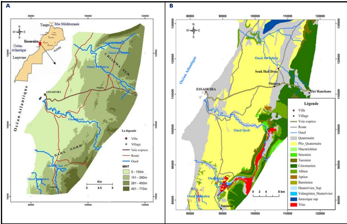
Fig. 1 - Contexte géographique et géologique de la zone côtière d'Essaouira. (A : Carte de localisation, B : Esquisse géologique).
