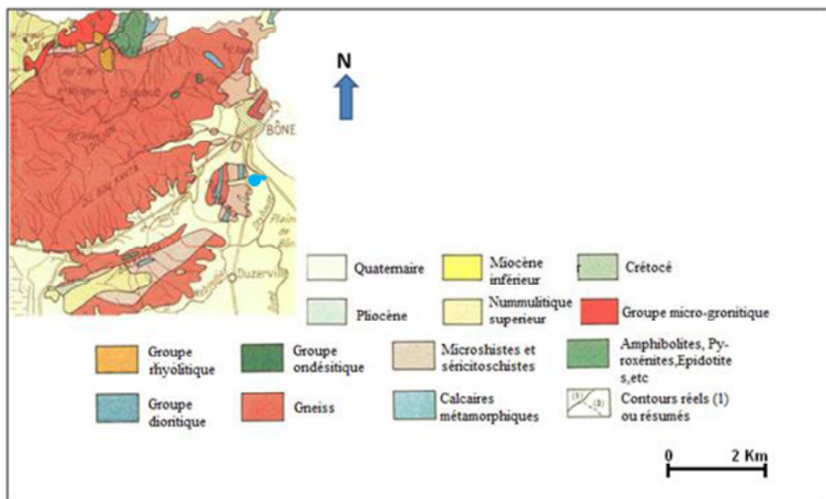
Fig. 2. Extrait de la carte géologique au 1/200 000 (Hilly, 1962)
