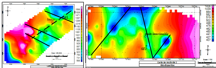
Fig. 2- Carte de résistivité apparente des sites 1 et 2
