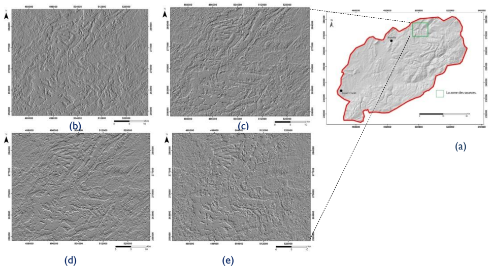
Figure 2 – Filtre de lissage appliqué sur la totalité du bassin (a). Filtres directionnels sur le couloir de cisaillement donnant naissance aux sources : filtre pour l'angle 0^{\circ} - 45^{\circ} (b), filtre pour l'angle 45^{\circ} - 90^{\circ} (c), filtre pour l'angle 90^{\circ} - 135^{\circ} (d), filtre pour l'angle 135^{\circ} - 180^{\circ} (e).
