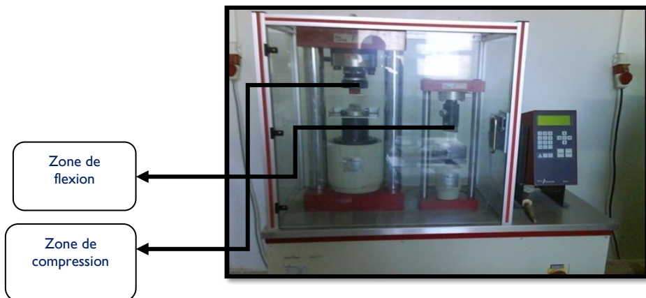
Figure 1. Appareil de flexion et de compression (Presse Toni Technik)
