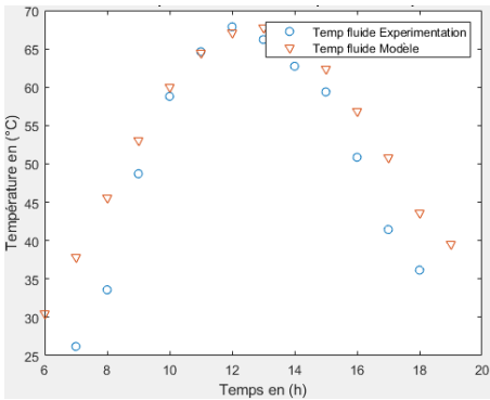
Fig. 6.b Temperature du fluide caloporteur
