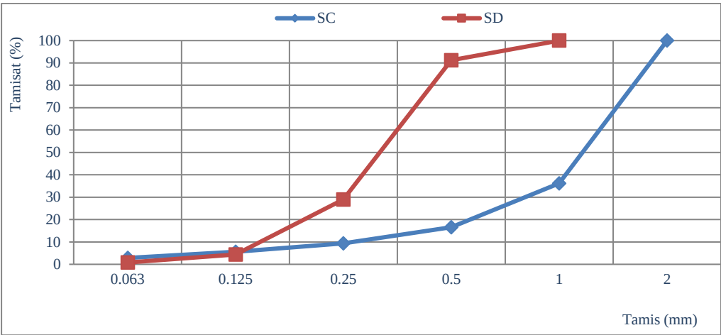
Fig. 1 – Courbe granulométriques des sables
