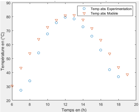
Fig. 6.a Temperature de l'absorbeur
