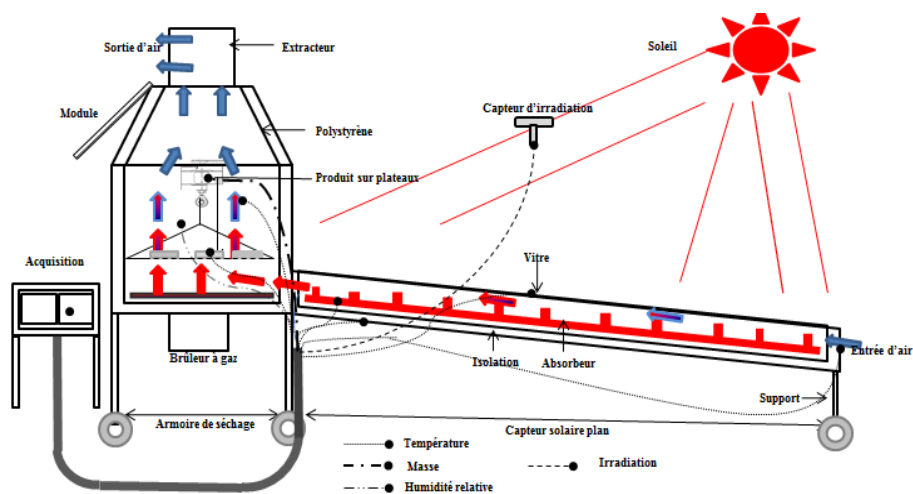
Fig. 1: Description du séchage solaire indirect
