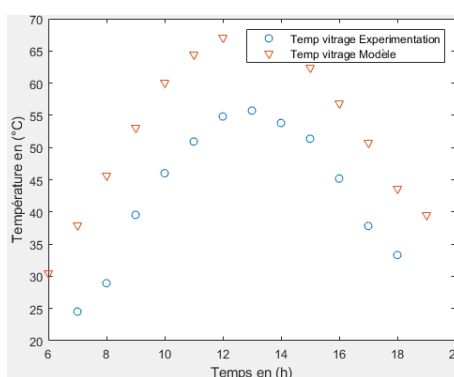
Fig. 6.d Temperature de la vitre face avant
