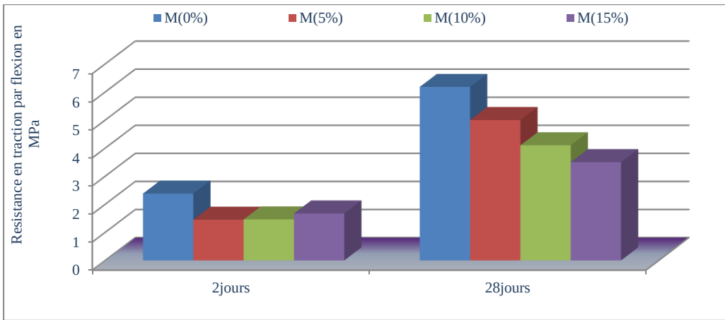
Fig. 6 - Influence du taux de substitution sur la résistance en traction par flexion
