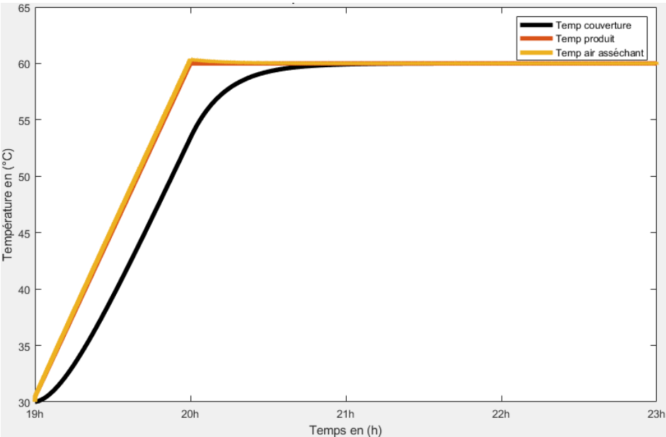
Fig. 5 : Températures de la couverture (interne et externe) et de l'air asséchant de l'unité de séchage en mode séchage à gaz
