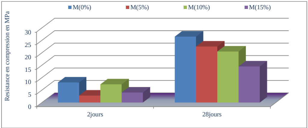
Fig. 5 – Influence du taux de substitution sur la résistance en compression
