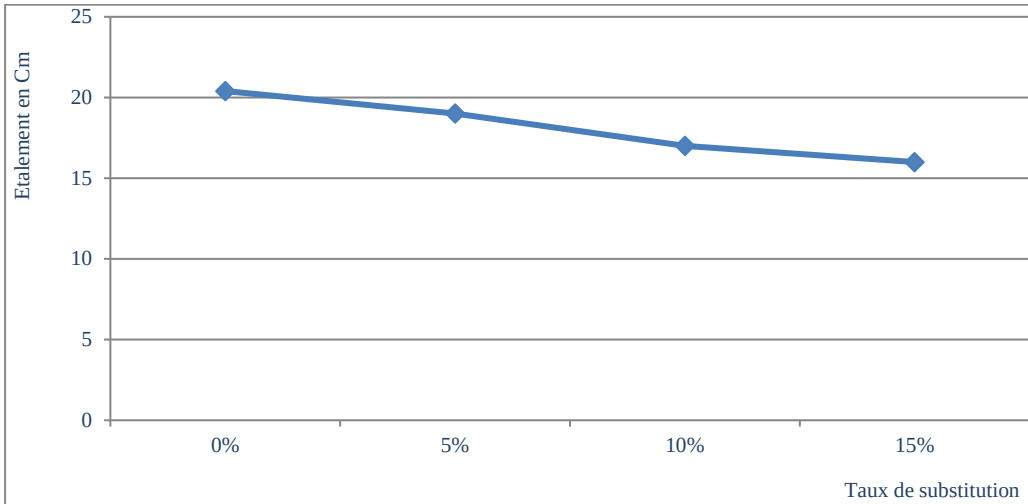
Fig. 3 - Variation de la consistance en fonction du taux de substitution
