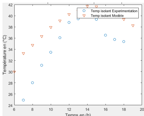
Fig. 6.c Temperature de l'isolant face arriere
