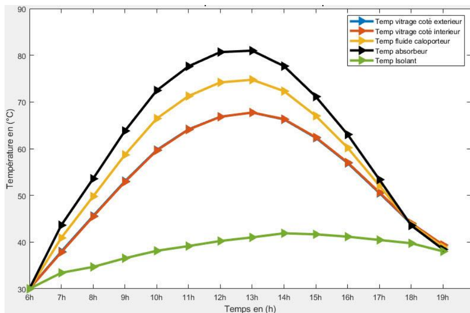
Fig. 3 : Températures des composants du capteur solaire
