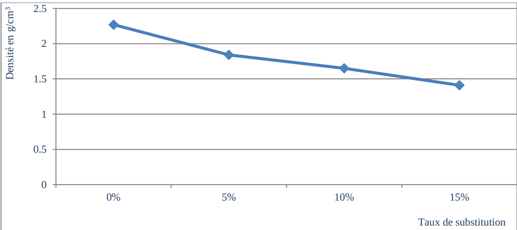
Fig. 2 - Variation de la densité en fonction du taux de substitution
