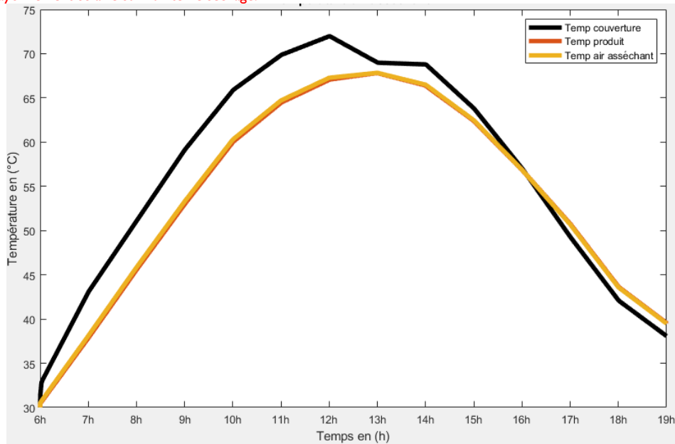
Fig. 4 : Températures de la couverture, du produit et de l'air asséchant de l'unité de séchage en mode séchage solaire indirect
