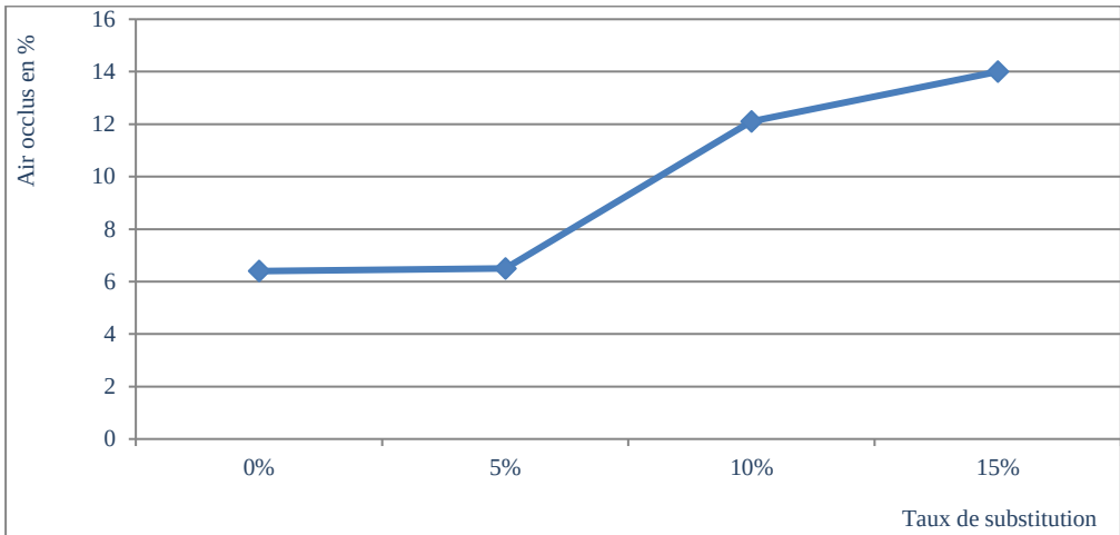
Fig. 4 - Variation de la teneur en air occlus en fonction du taux de substitution
