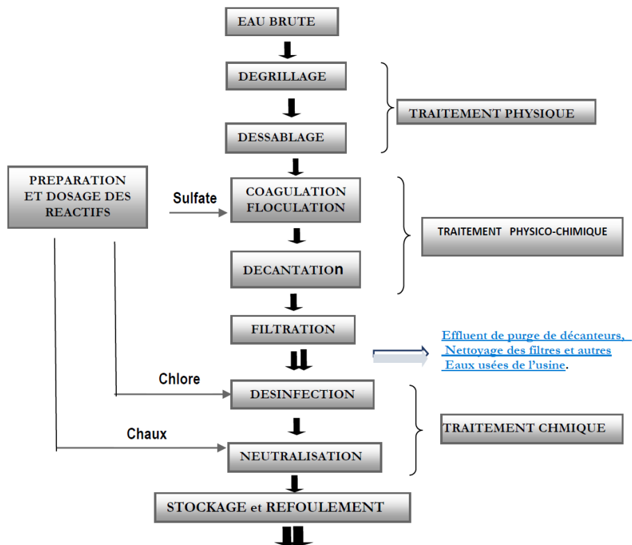
Figure I : Les étapes de traitement d'eau potable de l'usine de N'djili. (Source : Auteur, 2023).
