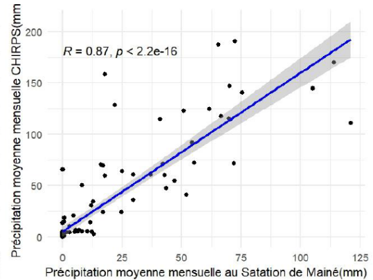
Figure 5 : Diagramme de dispersion des précipitations CHIRPS en fonction des précipitations in situ à la station de Mainé-Soroa, entre 2001 et 2010.
