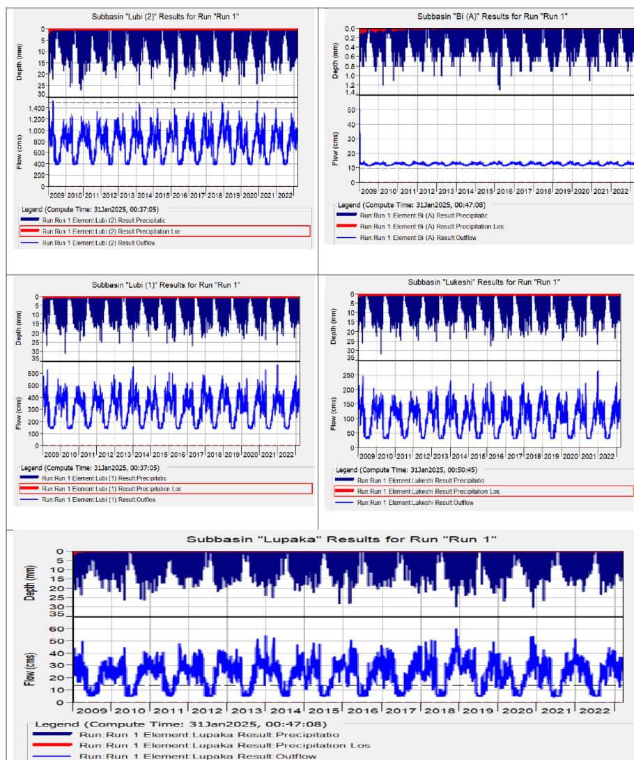
Figure3 : Simulation hydrologique de la Rivière LUBI
