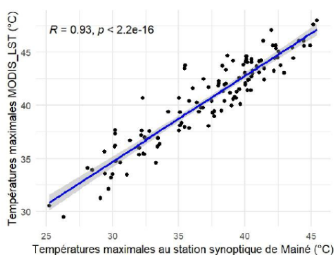
Figure 3 : Diagramme de dispersion des températures MODIS_LST en fonction des températures in situ à la station de Mainé-Soroa, entre 2001 et 2010.
